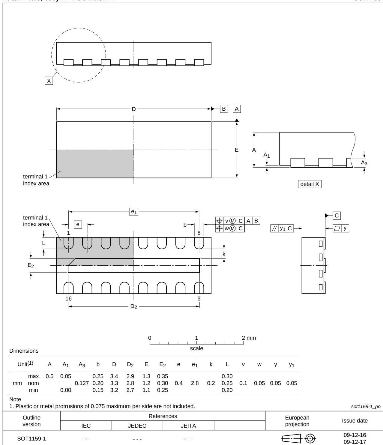
Fig 12. Package outline PEM18QFN (SOT1159-1/HXSON16)
